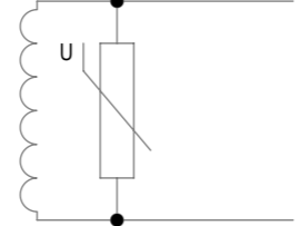
el. Schaltbild mit Löschiglied / circuit diagramm with suppressor
